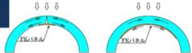
当て板工
